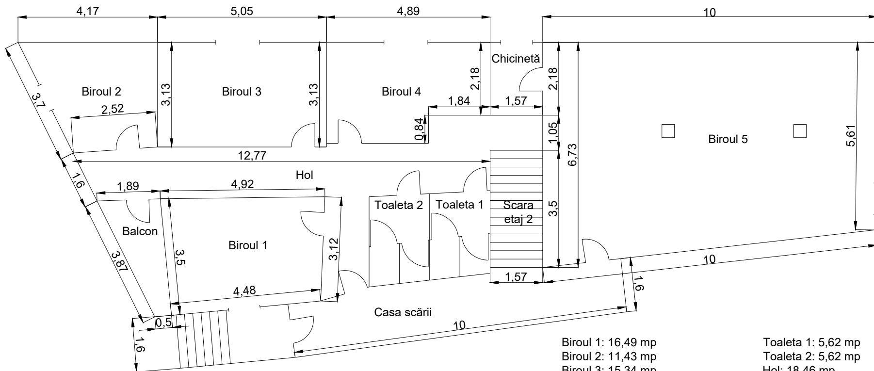
Plan Etaj 1
