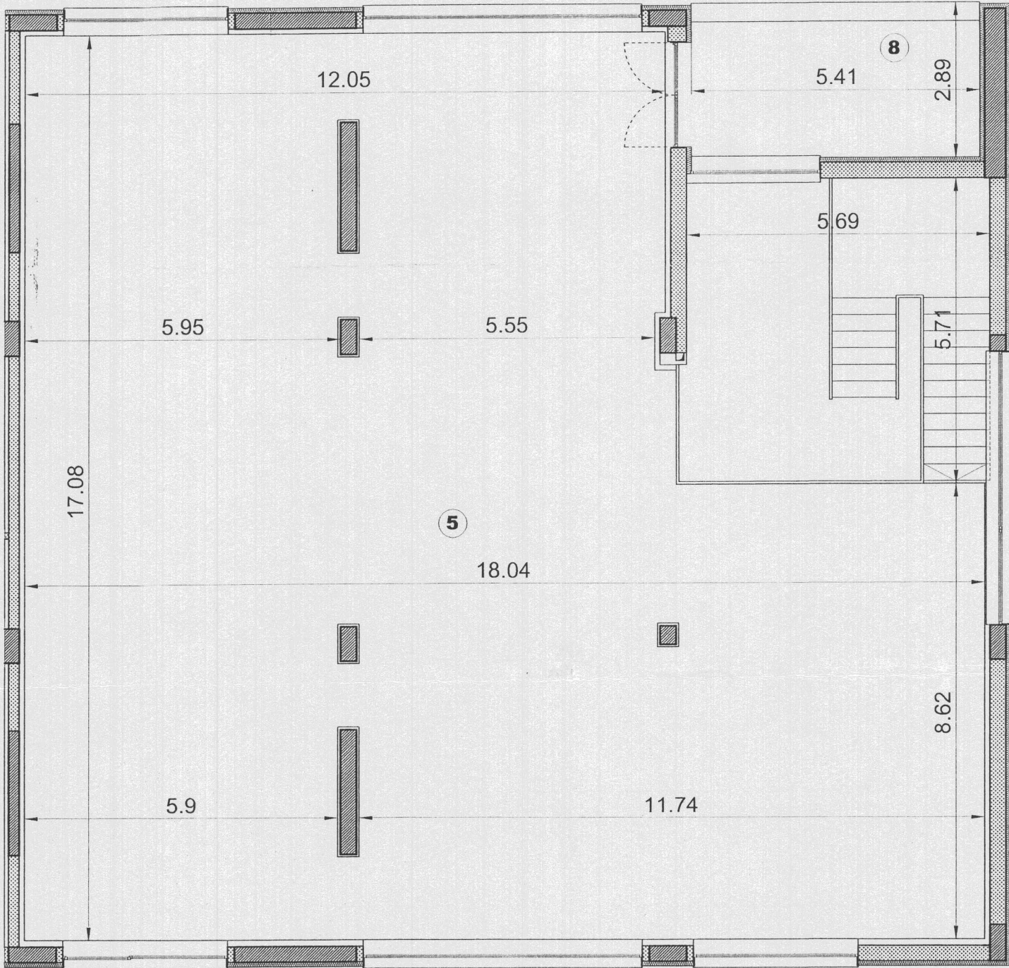
ETAJ GRADINITA
